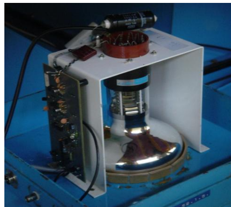
Figura 32: Fotomultiplicadora
